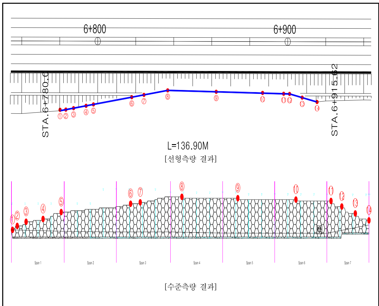
【그림 11.3.5】 선형 및 수준측량 결과
